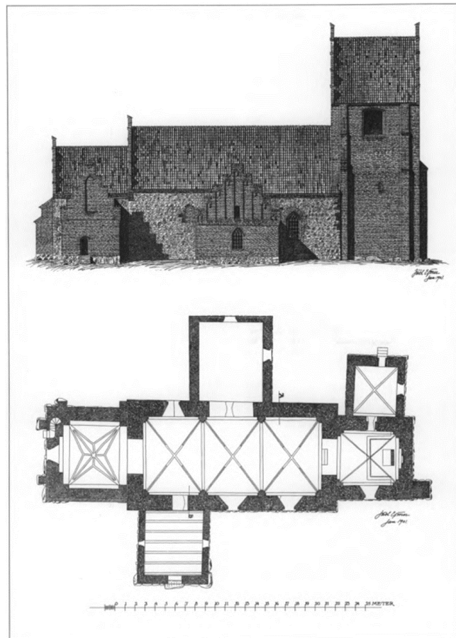
Opmåling af kirken fra 1901. Plan og facade mod nord
